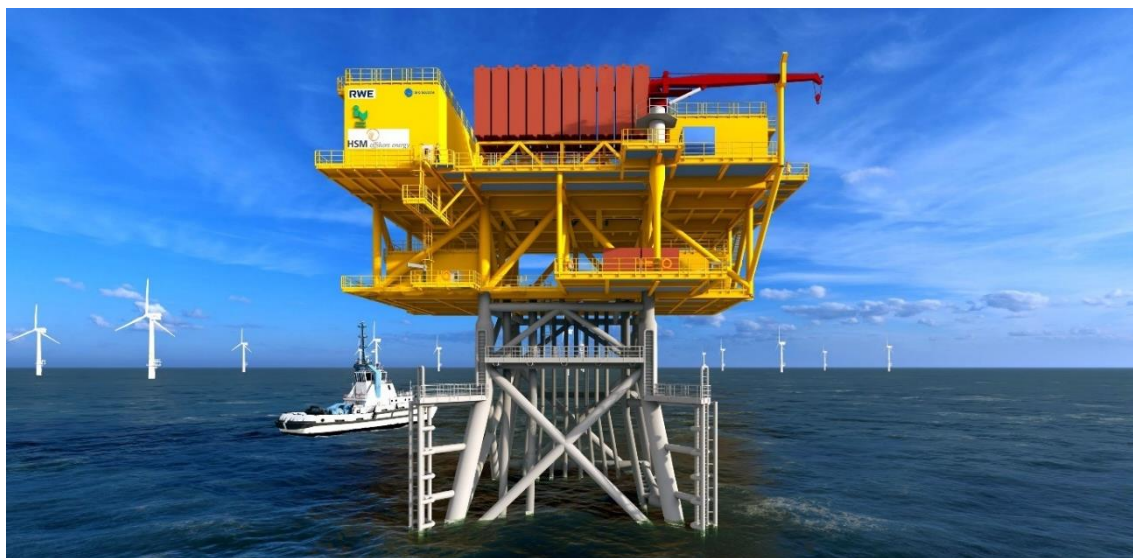
Figur 18. Illustration av transformatorstation på fackverksfundament för Thor vindpark 1060 MW, Danmark, (RWE).
