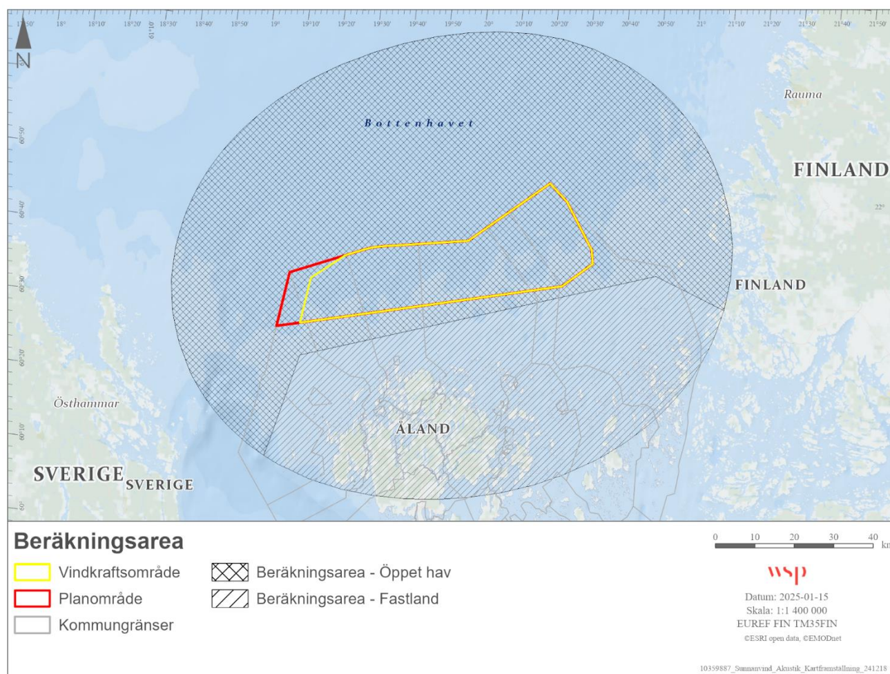
Figur 7. Areor för beräkning av ljudnivåer från vindkraftsparken.
