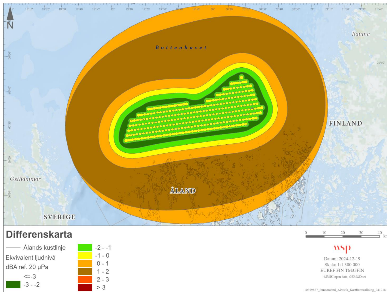
Figur 15. Differensskarta som visar skillnaden i ljudnivå mellan medvind och motvind.
